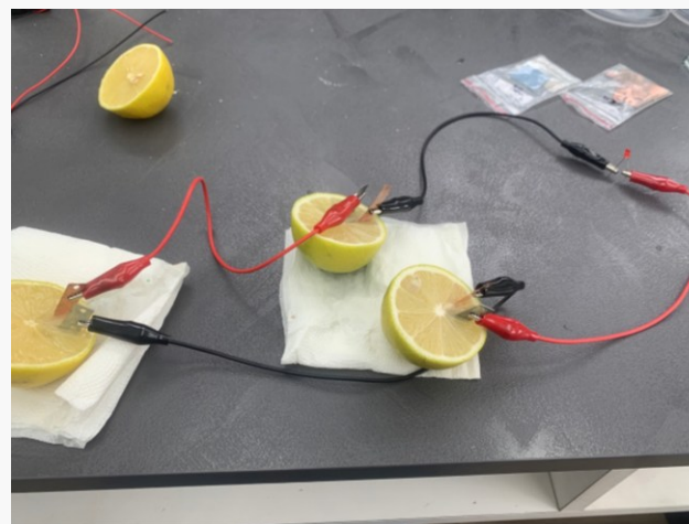
三顆發光，但微弱， 實驗三可測試串聯更多個。
